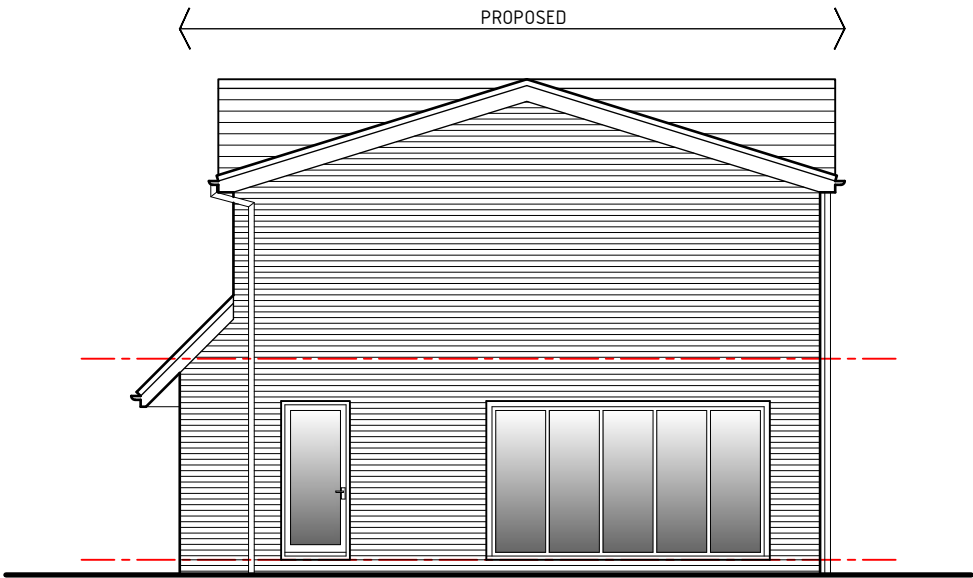
Side-02 elevation 1:100
