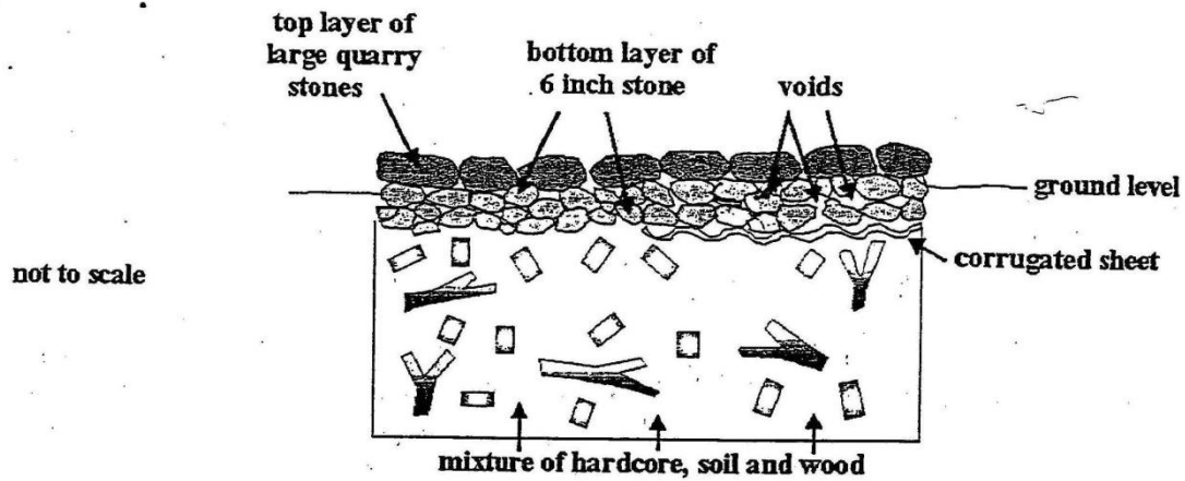
LONGITUDINAL SECTION
