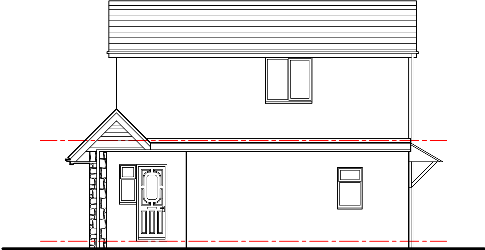
Side-02 elevation 1:100
