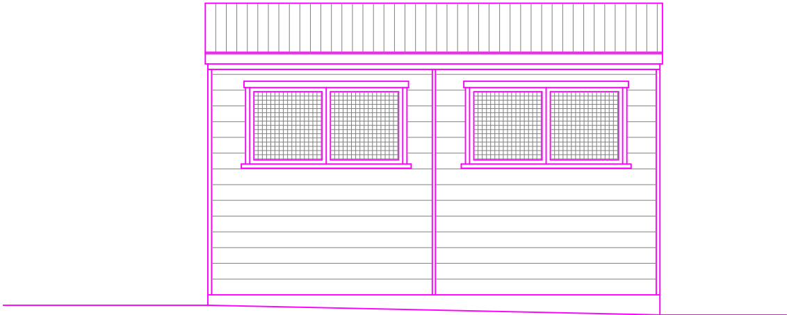
Side-01 elevation 1:50
