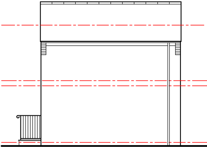
Side-02 elevation 1:100
