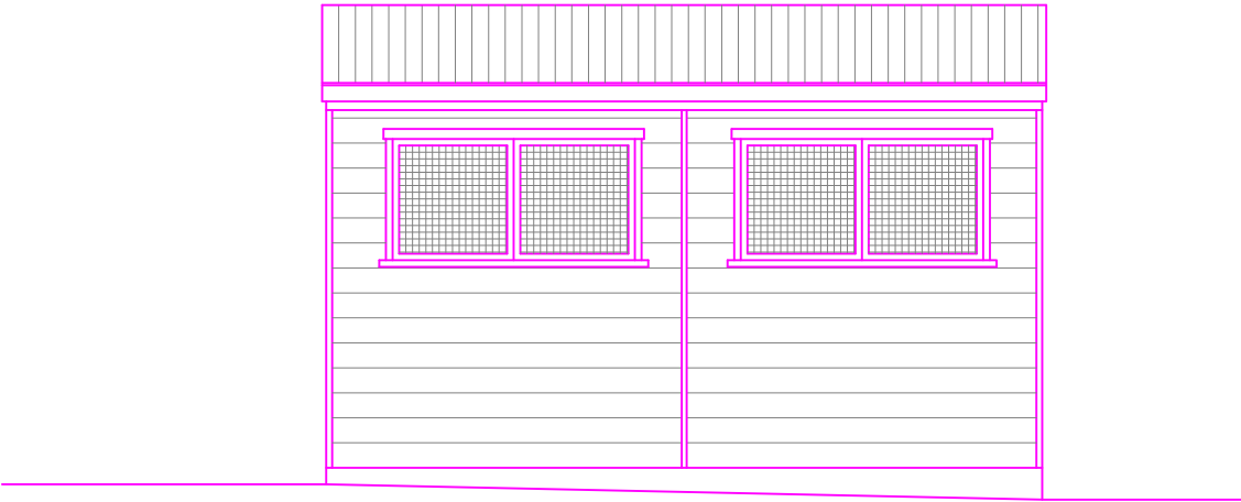
Side-01 elevation 1:50
