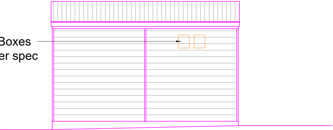
Side-02 elevation 1:50
