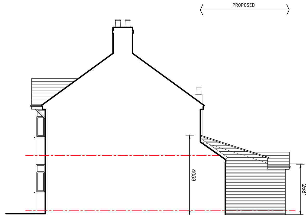
Side-02 elevation 1:100
