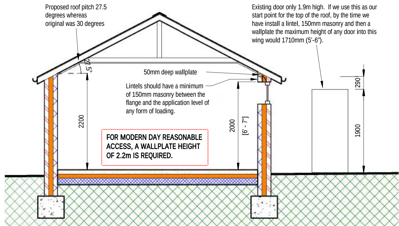
SECTION A-A
