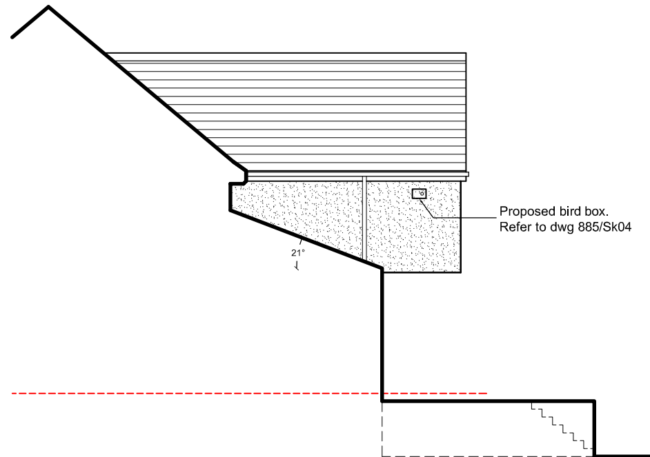
RETURN ELEVATION
