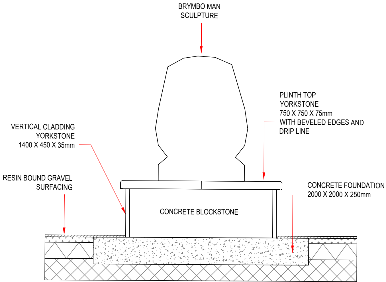
23 1:20 BRYMBO MAN - YORKSTONE PLINTH
