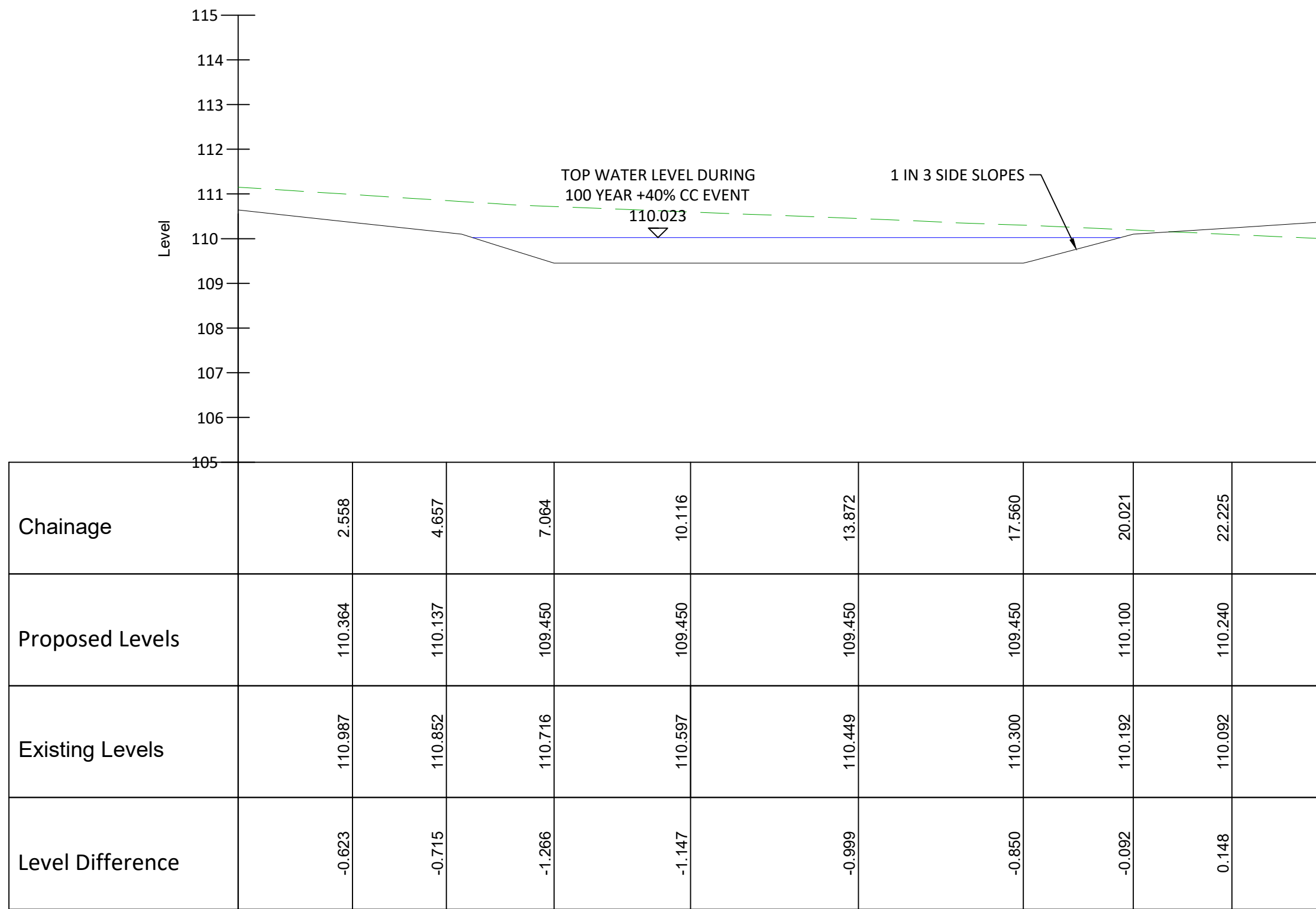
SECTION A-A 1:100
