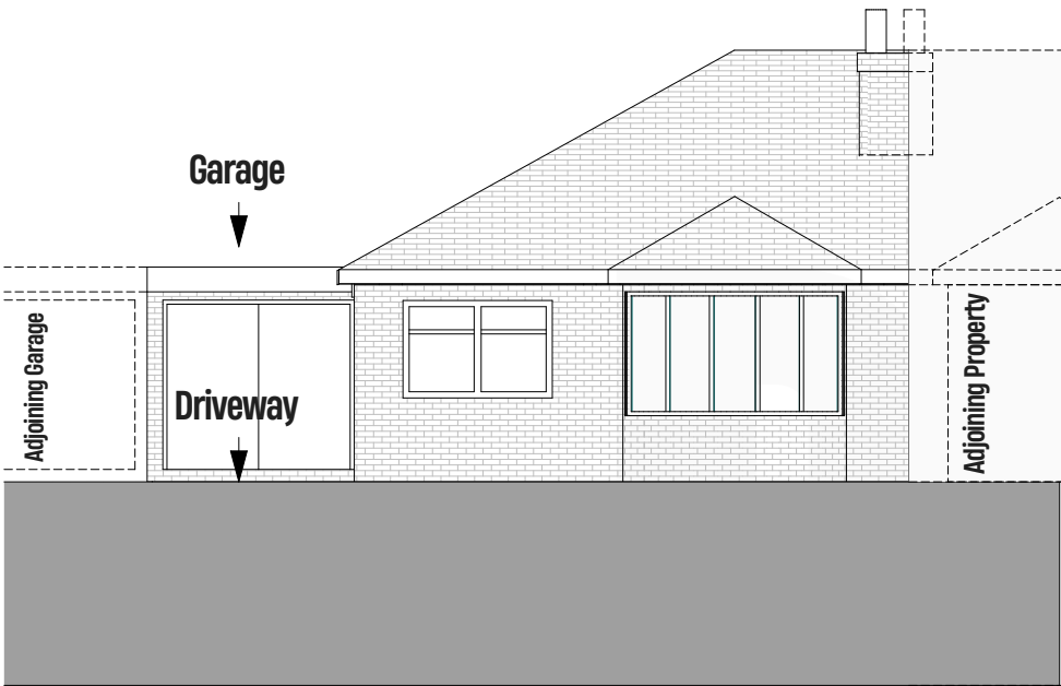
E1 Front Elevation 1:100
