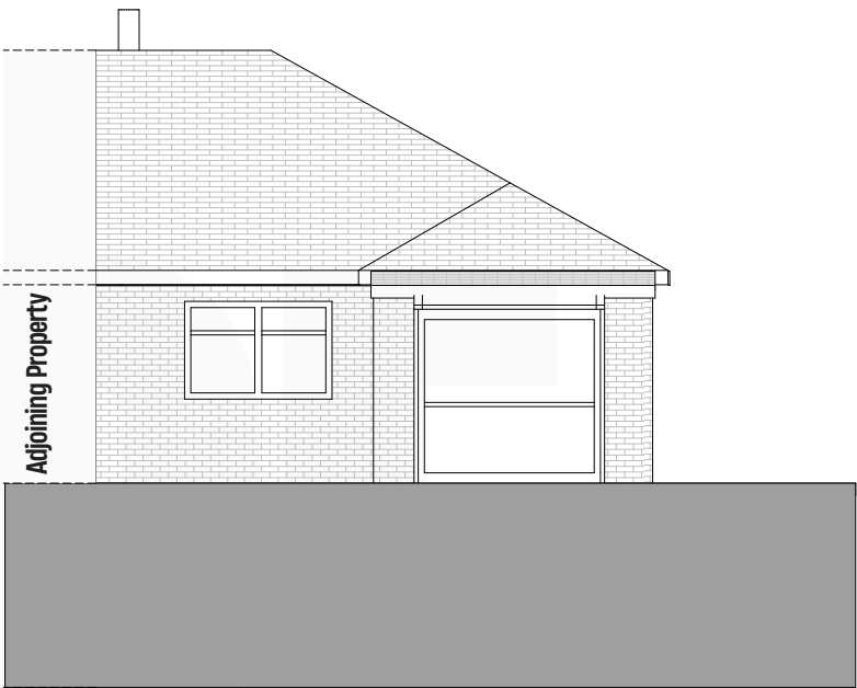
E3 Rear Elevation 1:100
