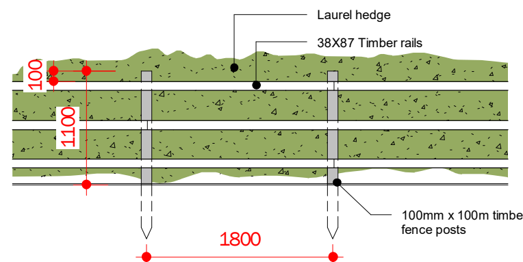
F2 - Field Fence Scale: 1:50
