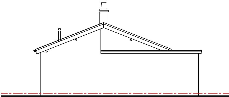
Side-02 elevation 1:100
