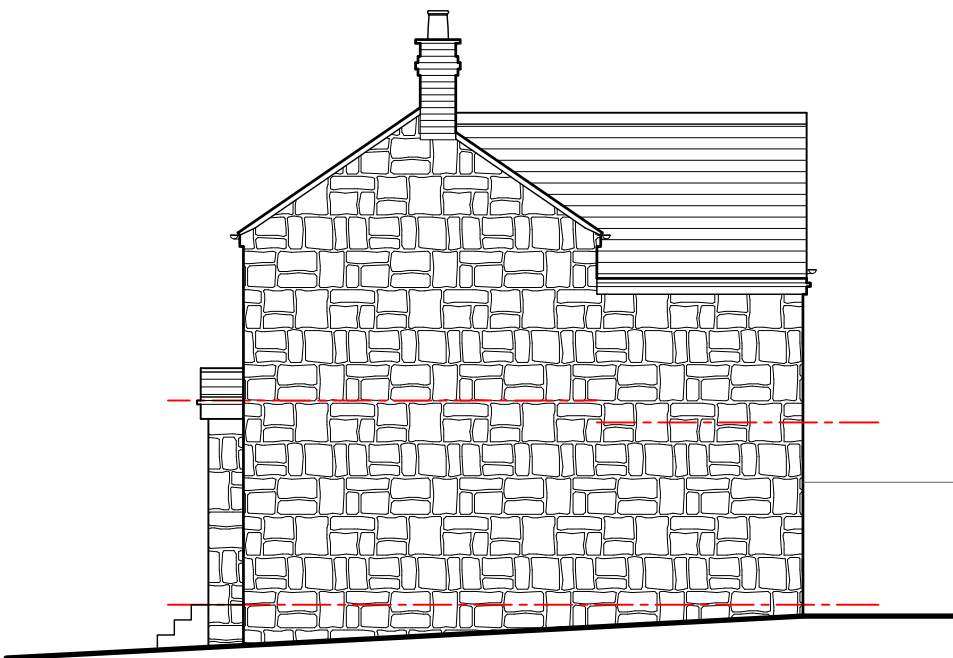
Side-02 elevation 1:100
