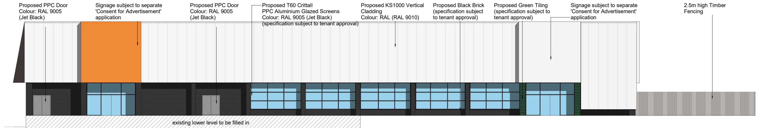
West 1 : 100
