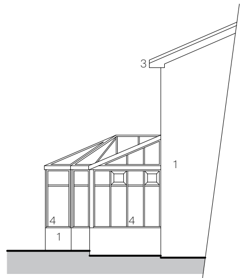
Side Elevation Scale: 1:100
