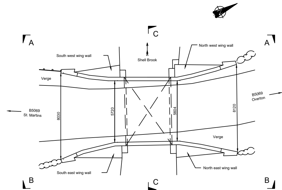
PLAN Scale 1 : 100
