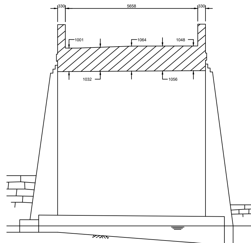
SECTION C - C Scale 1 : 50
