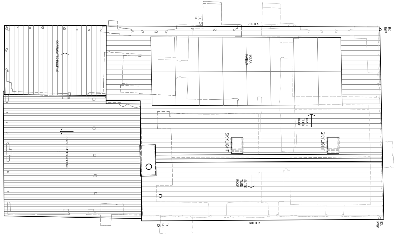
roof plan 1 : 100
