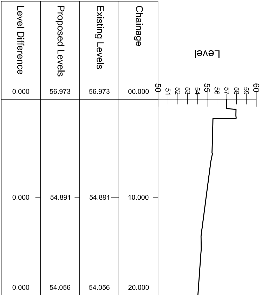
SITE SECTION 18 - LONGSECTION SCALE: H 1:100, V 1:100, DATUM: 50.000
