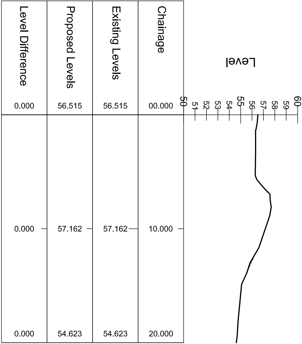
SITE SECTION 17 - LONGSECTION SCALE: H 1:100, V 1:100, DATUM: 50.000
