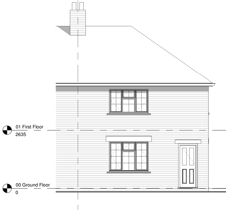
Existing SE Elevation 1 : 50
