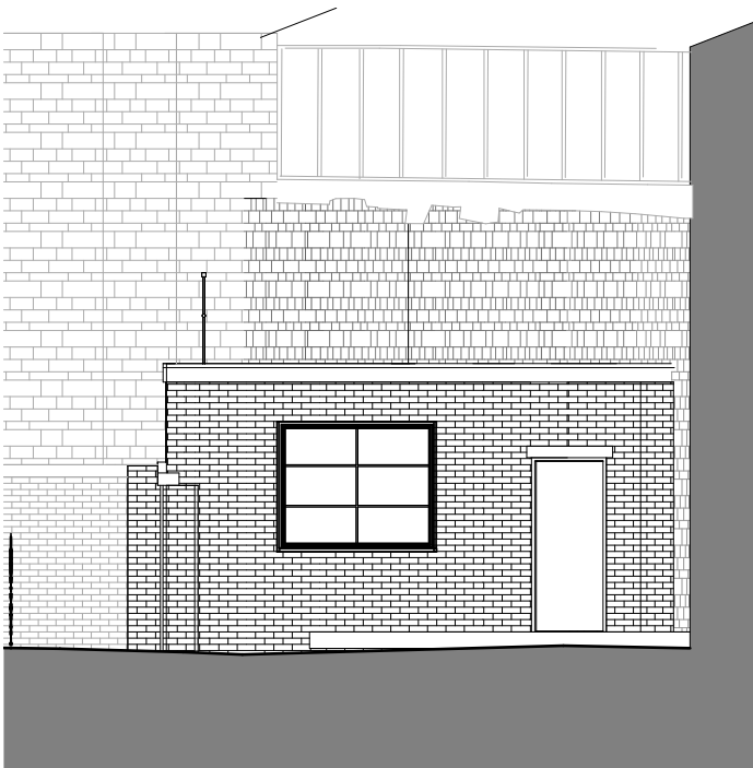
Side Elevation 01 1 : 100
