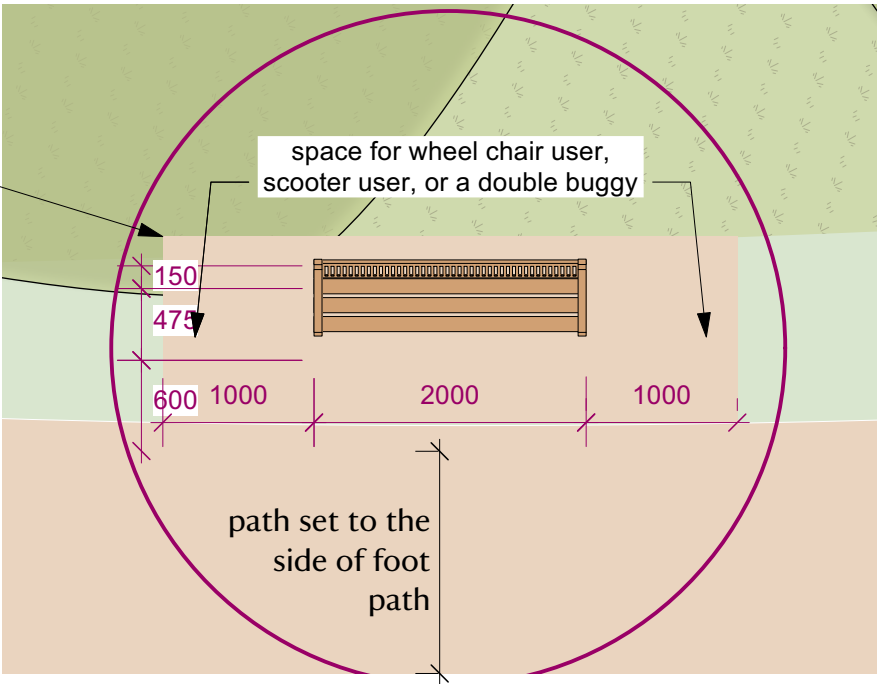
Plan - 1:50
