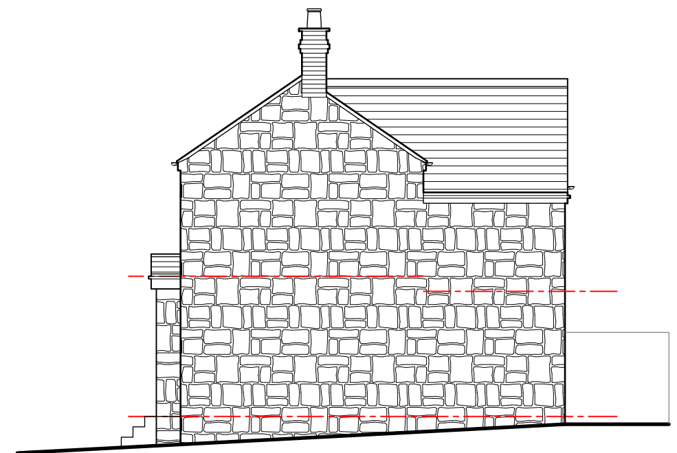
Side-02 elevation 1:100
