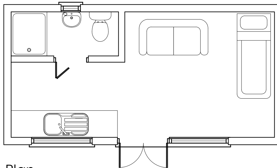
Plan 1:50
