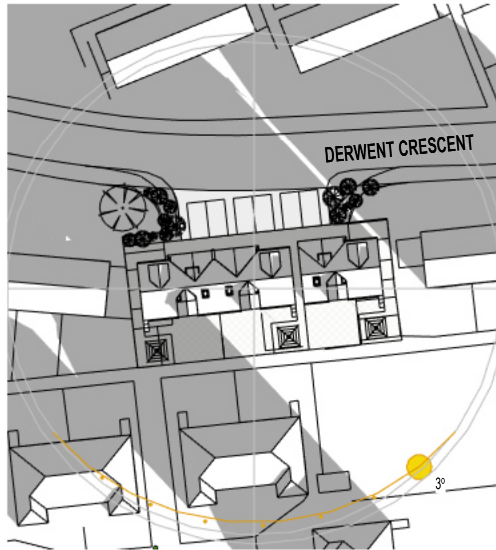
4 Dec 21 0900 1 : 500 Winter Solstice sunrise 08:04 sunset 15:53
