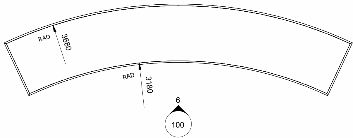
Besoke Stone Bench - Plan 1 : 20
