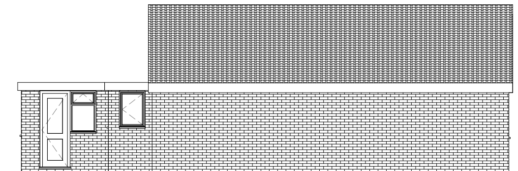
3 East 1 : 100
