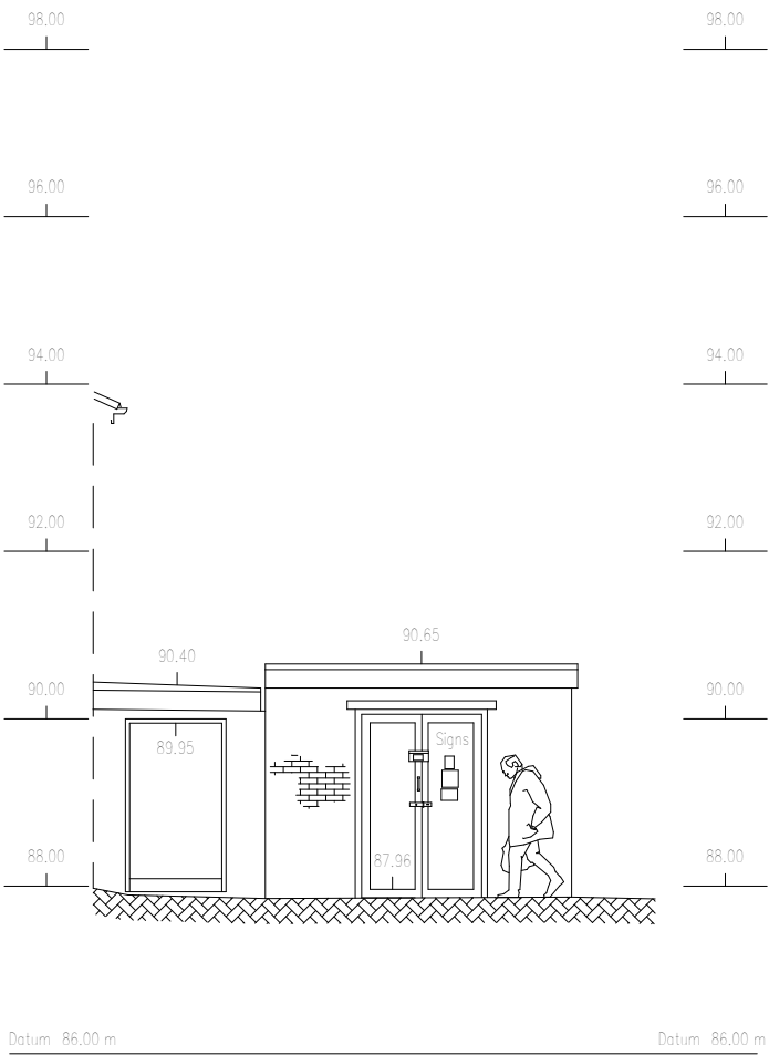
Elevation J
