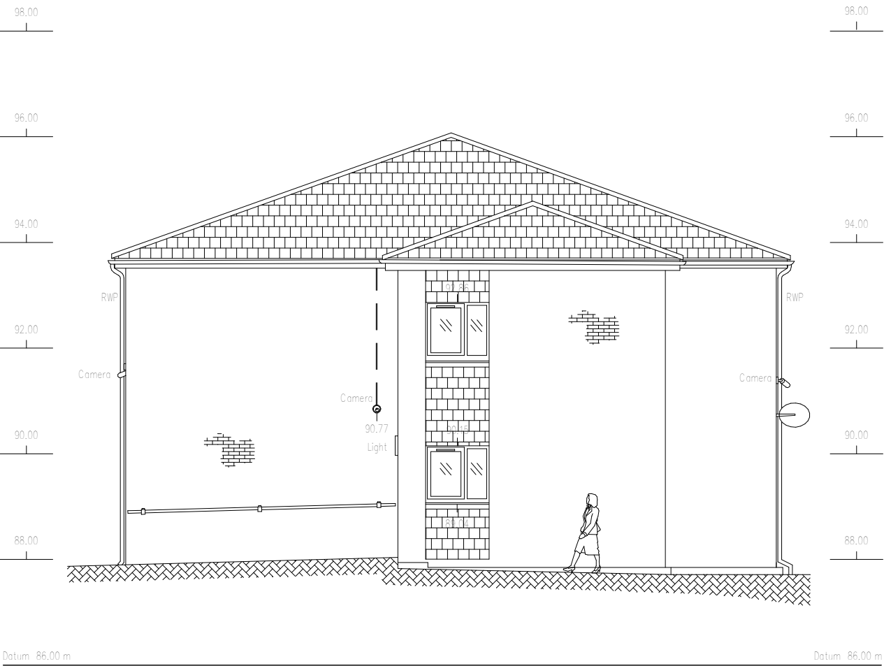
Elevation G
