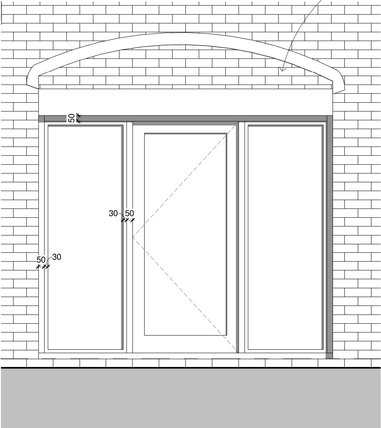
New Entrance Door 1 : 20
