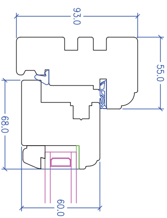
Window Typ. Jamb
