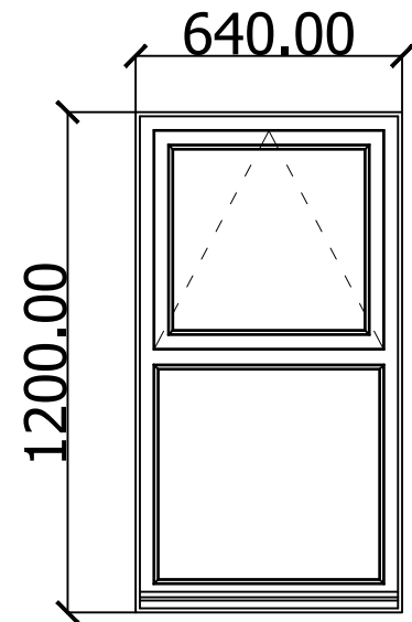
Elevation
