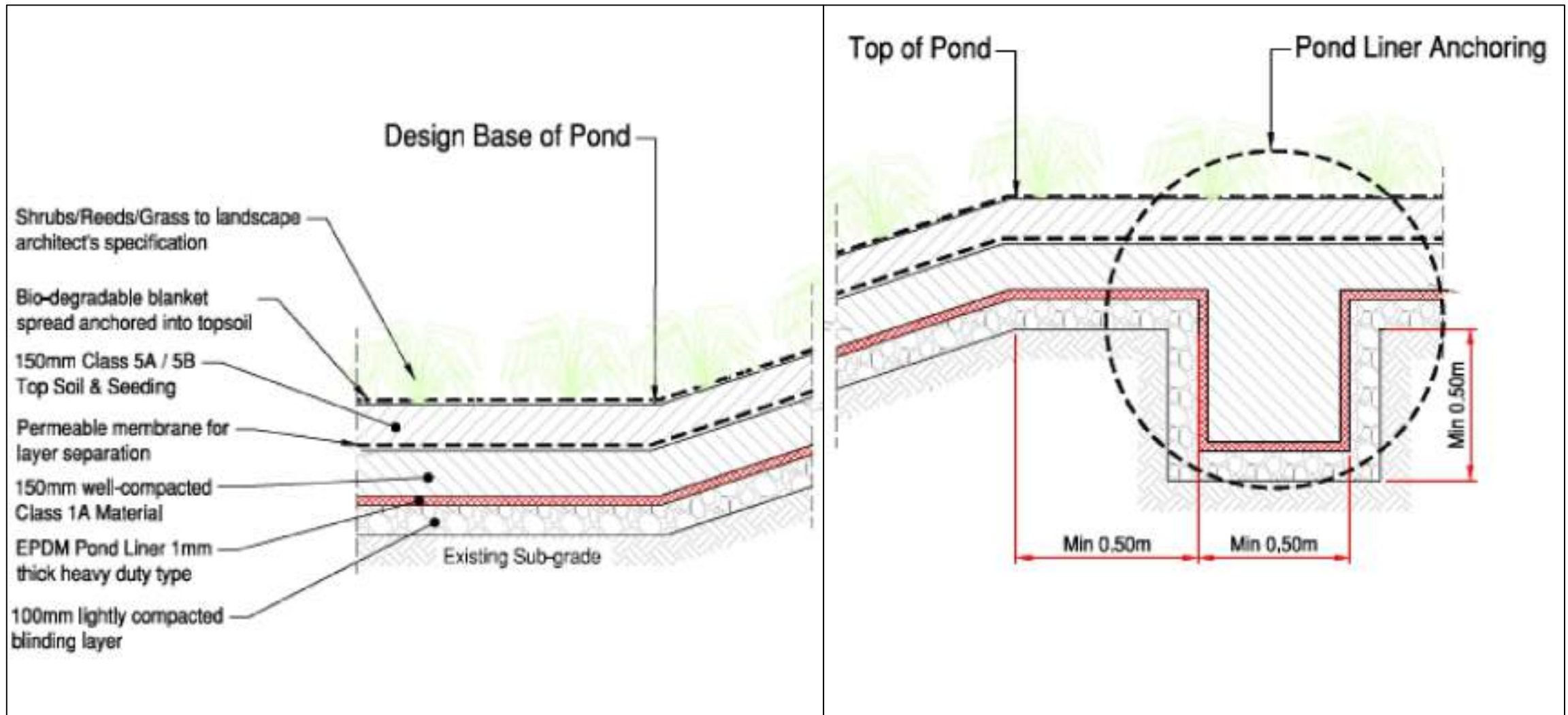
Insert A Pond Construction Details (N.T.S)
