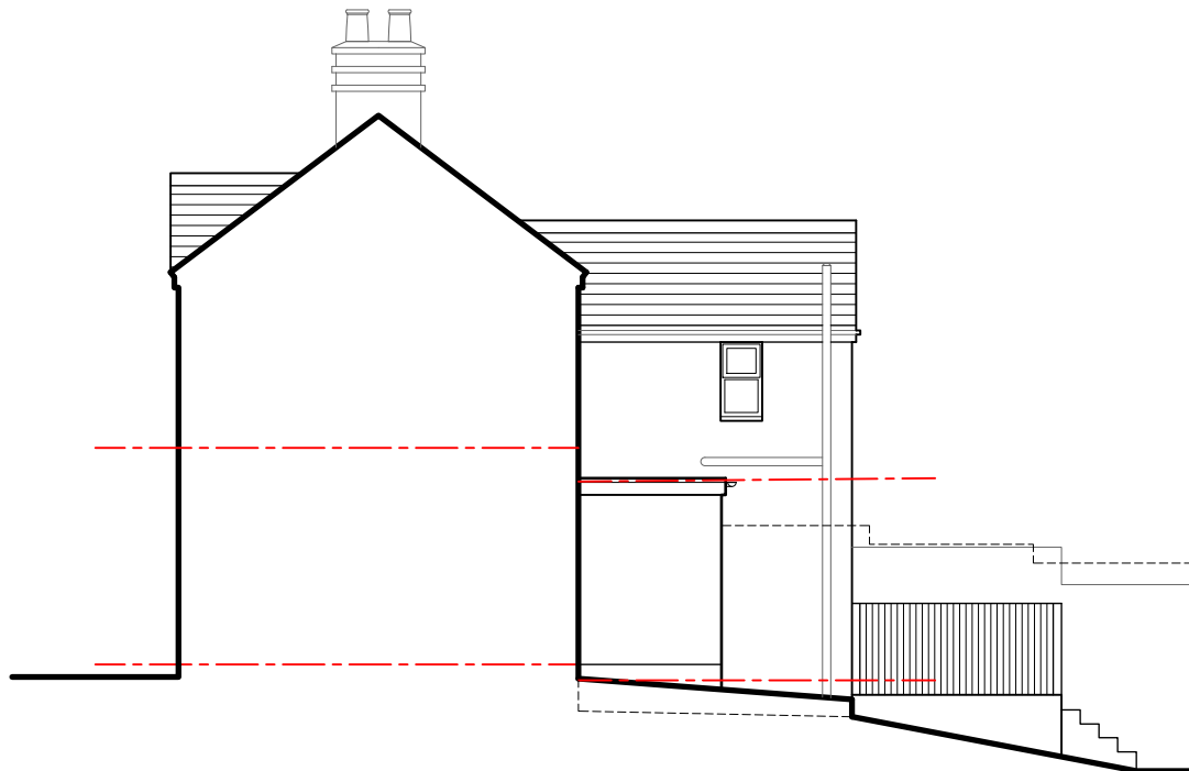
Side-02 Elevation 1:100
