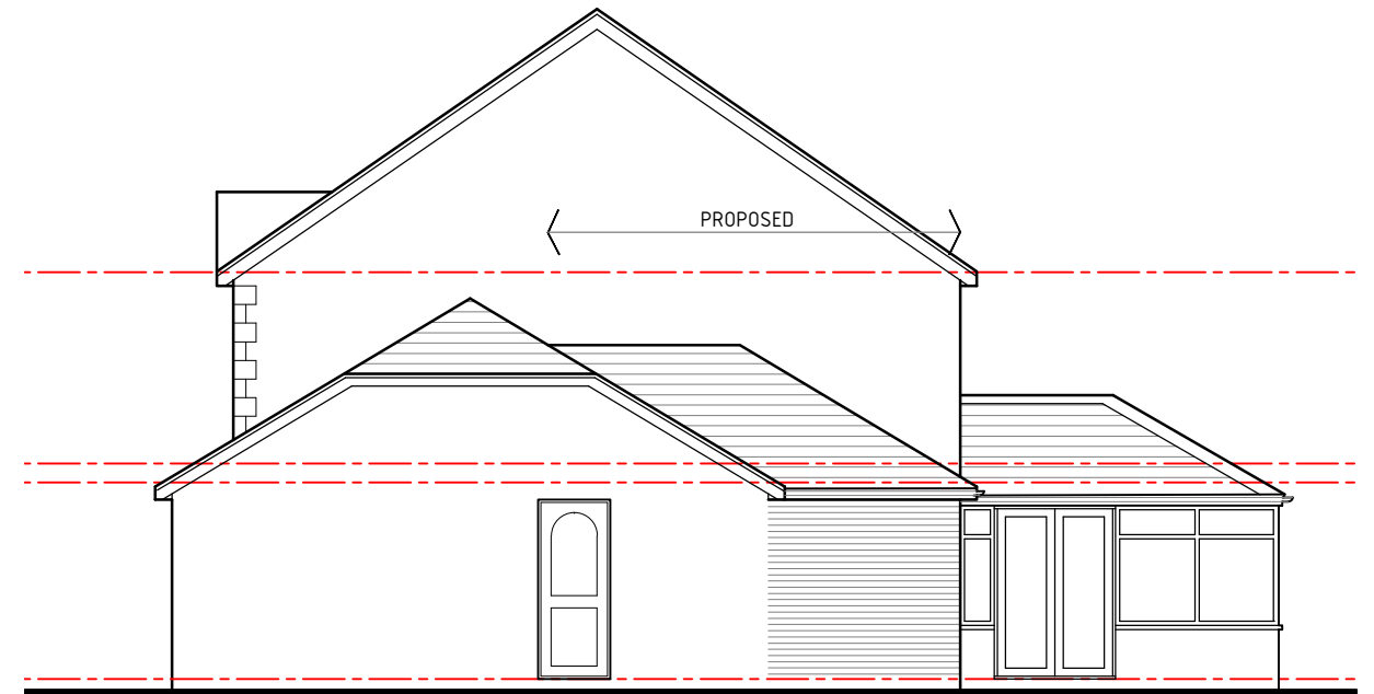
Side-02 Elevation 1:100
