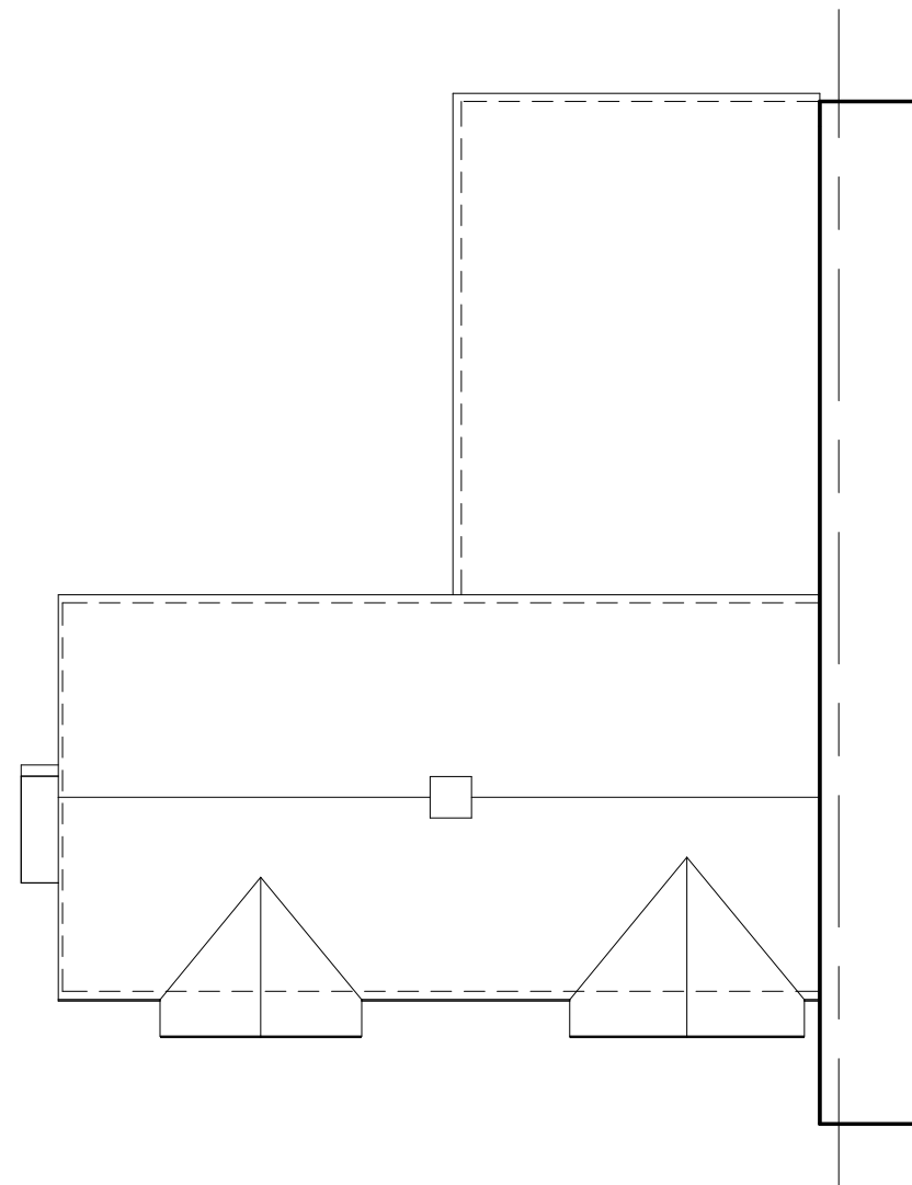
Roof Plan 1 : 100
