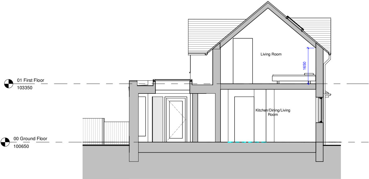
Section B-B 1 : 50 (1 : 100 @ A3)
