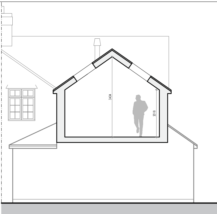
Rear Section Scale: 1:100
