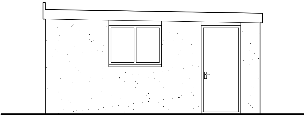
Side-02 elevation 1:50
