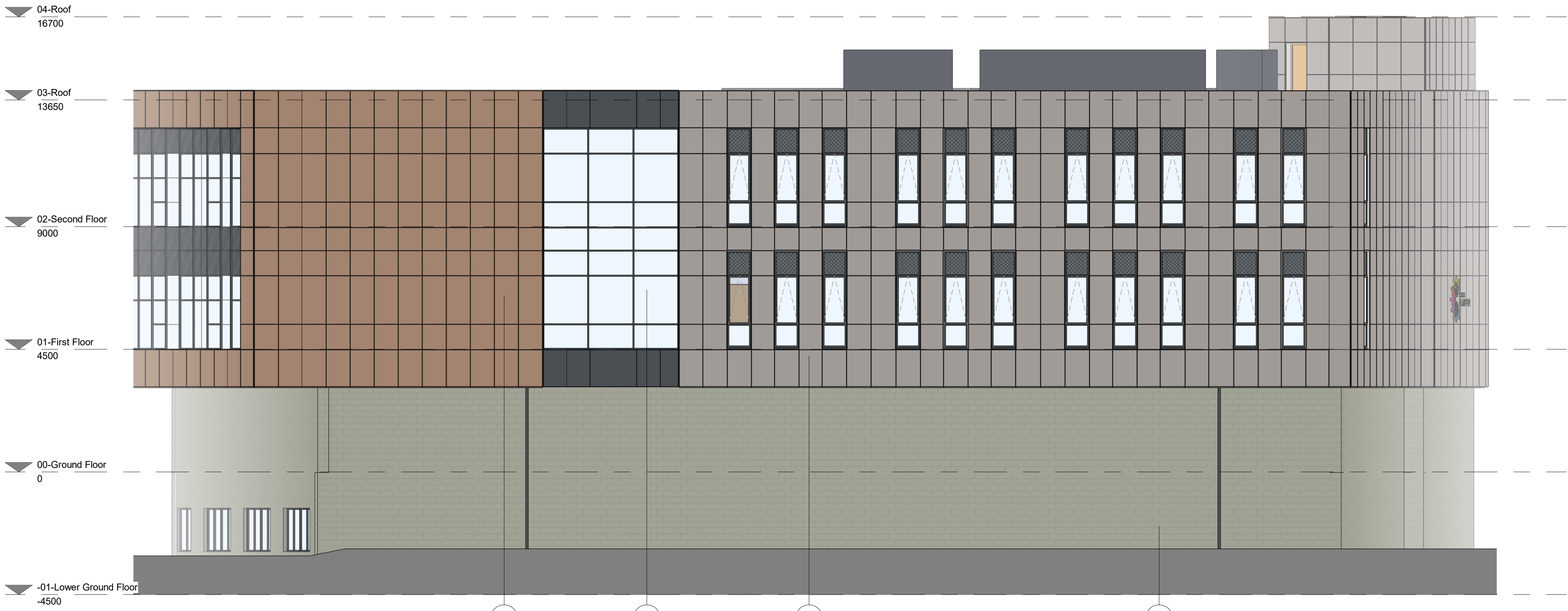
6 GA Elevation 6 1 : 100
