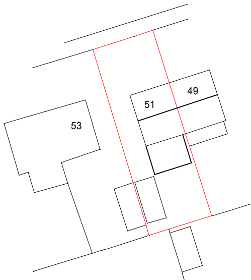
SITE PLAN 1:500
