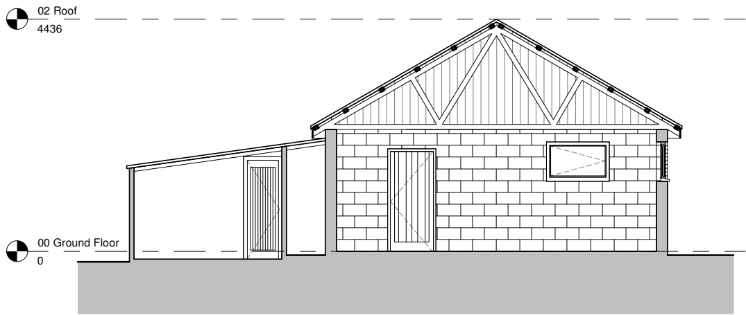
Section A-A 1 : 50
