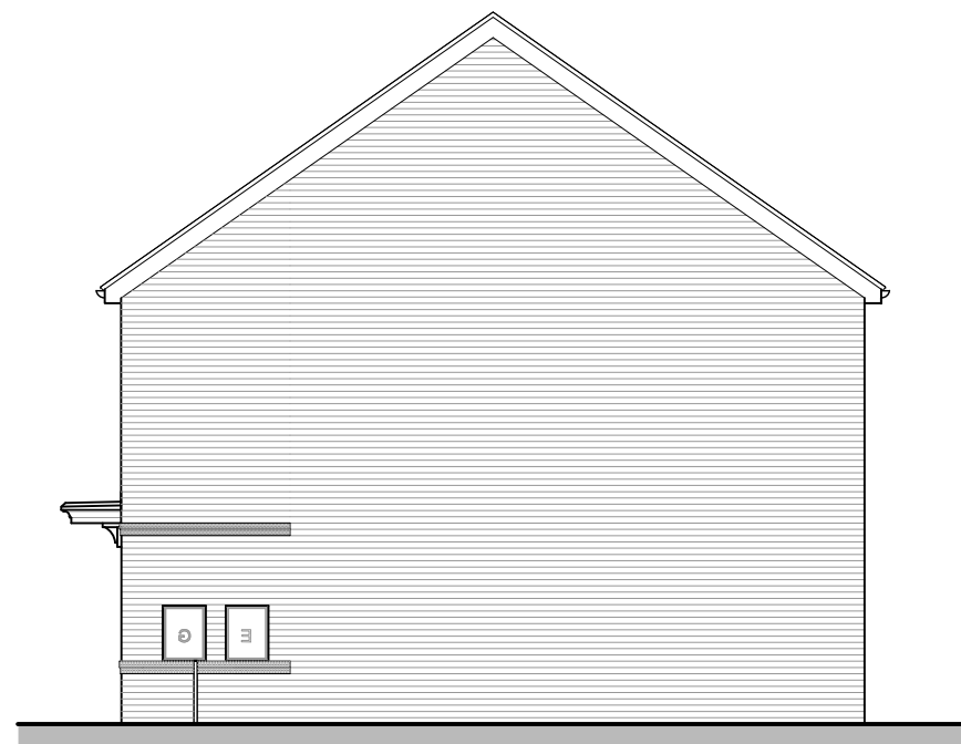
CLWYD END OPP SIDE ELEVATION
