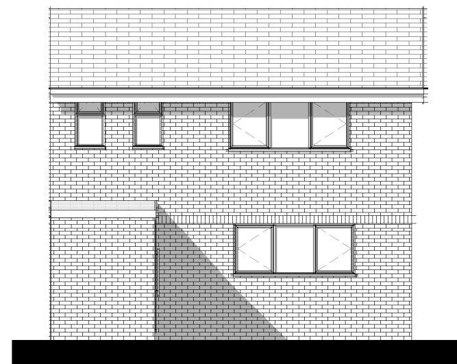
WEST _____ 1 : 100
