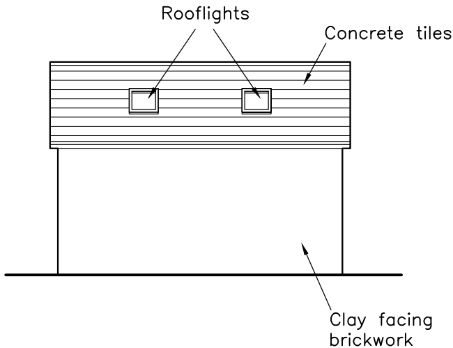
ELEVATION 3
