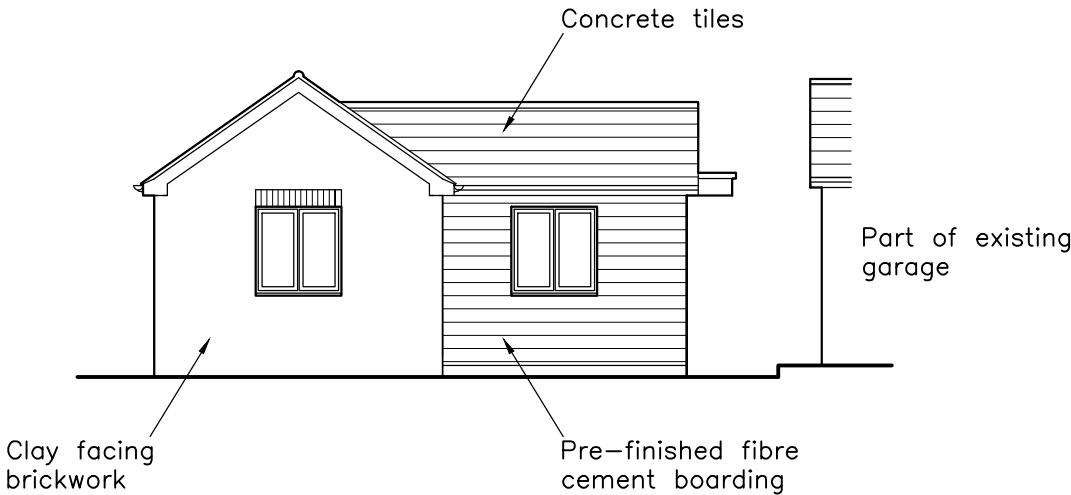
ELEVATION 2
