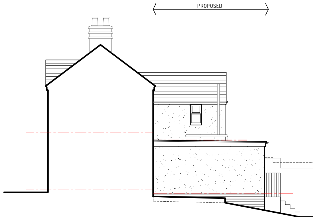
Side-02 Elevation 1:100
