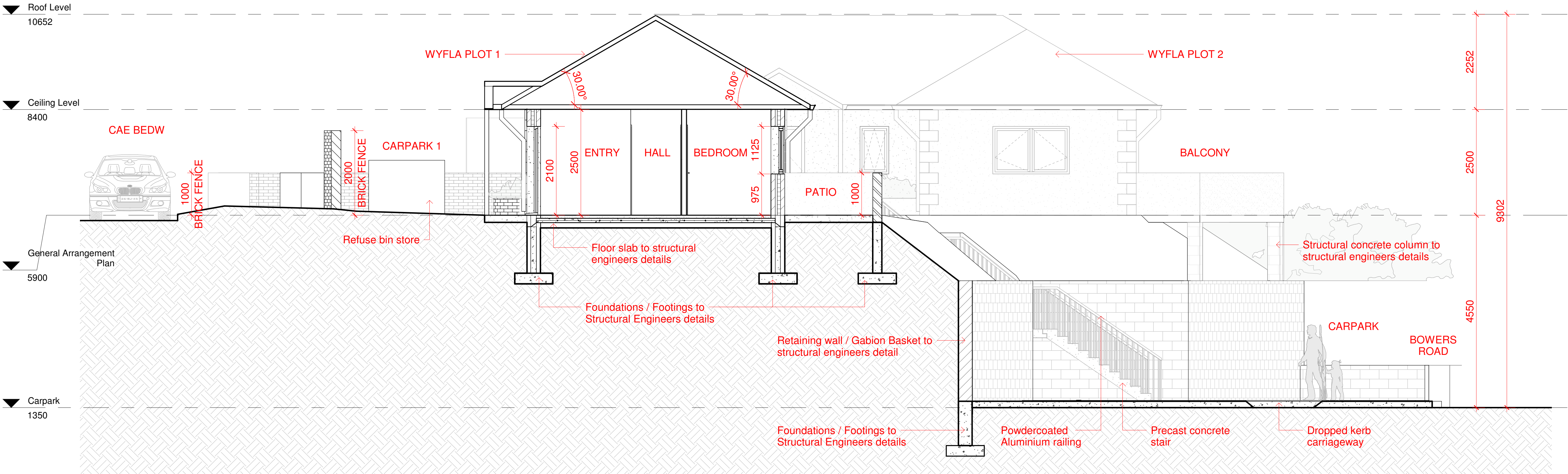
1 Site Cross Section 1 : 50
