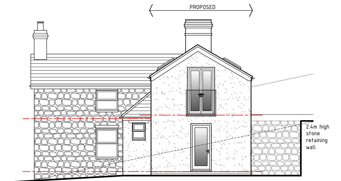
Side-02 elevation 1:100
