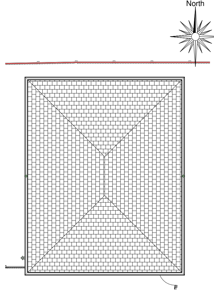
5 Roof Plan 1 : 100
