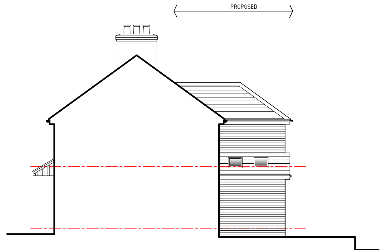
Side-02 elevation 1:100
